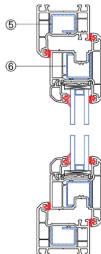
纵向节点图
