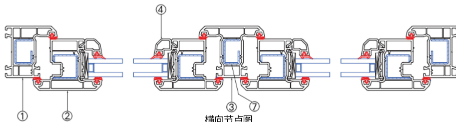
横向节点图
