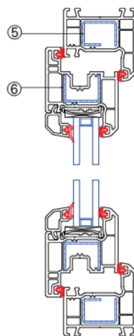
纵向节点图
