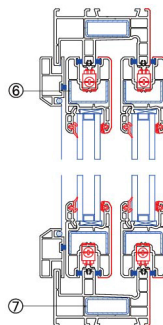
纵向节点图
