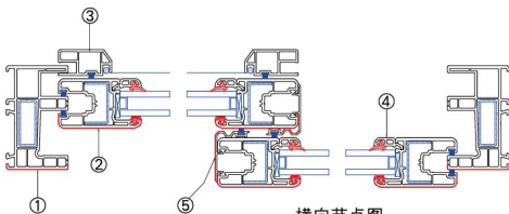
横向节点图
