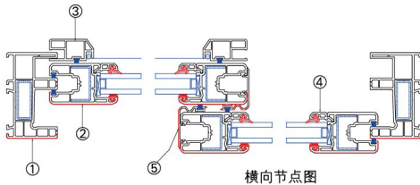
横向节点图
