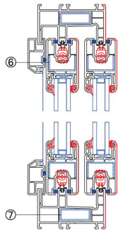
纵向节点图
