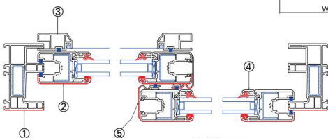
横向节点图
