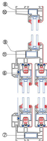
纵向节点图
