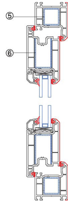
纵向节点图
