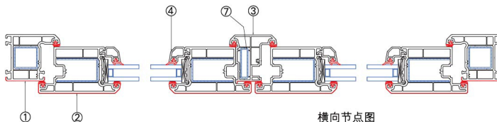
横向节点图
