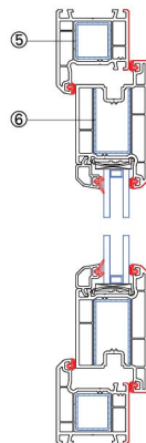
纵向节点图
