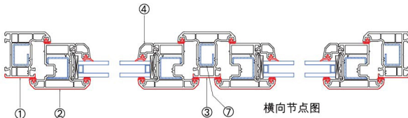
横向节点图
