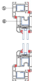
纵向节点图
