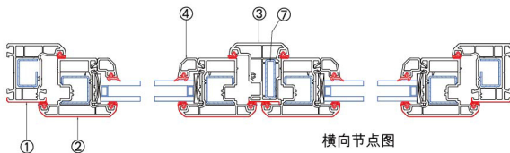
横向节点图
