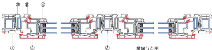
横向节点图
