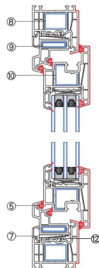
纵向节点图
