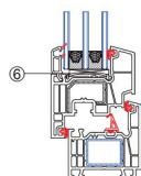
纵向节点图
