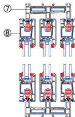
纵向节点图
