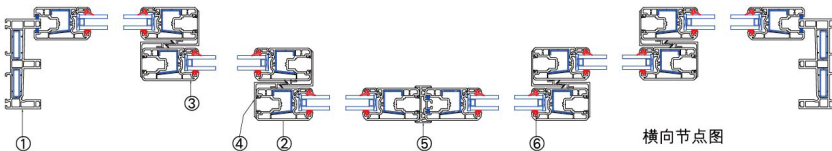
横向节点图
