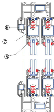
纵向节点图
