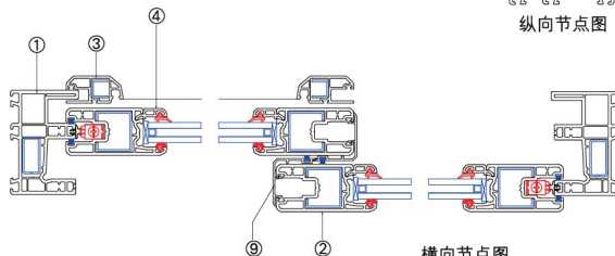
横向节点图
