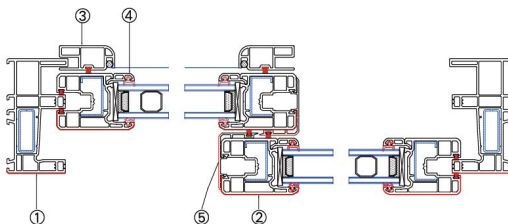
横向节点图
