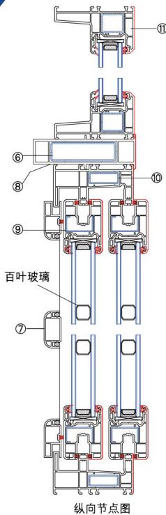
纵向节点图
