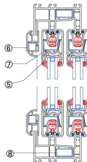
纵向节点图
