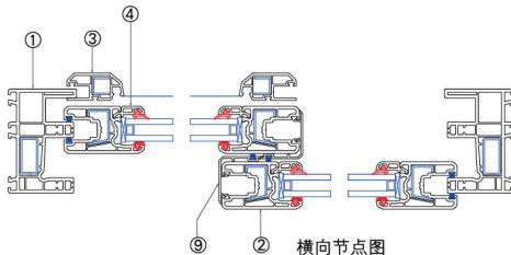
横向节点图
