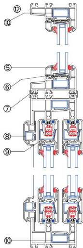
纵向节点图
