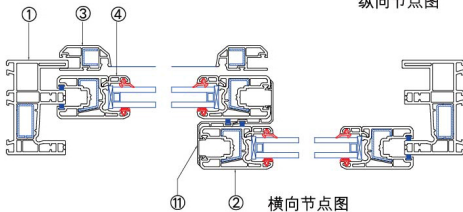
横向节点图
