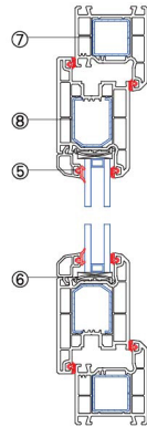
纵向节点图
