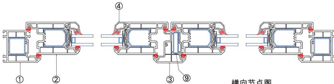
横向节点图
